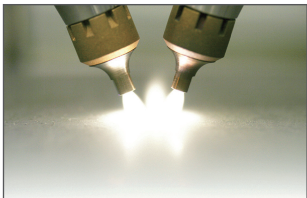
Plasmabeam Duo double nozzles system Plasmabeam Duo Doppeldüsenanordnung
